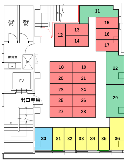
6階平面図
