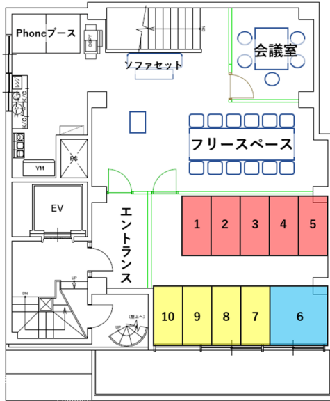
7階平面図
